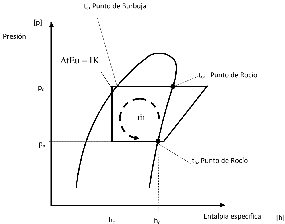
Fig.1: Diagrama Presión-Entalpía
